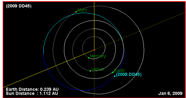
Орбита астероида 2009 DD45). Изображение http://www.spaceweather.com с сайта http://www.astroalert.su
