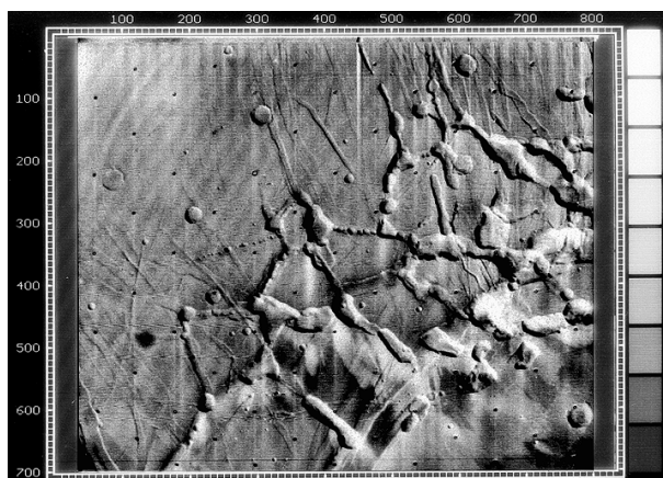
Фотография поверхности Марса с аппарата «Маринер-9». Изображение с сайта http://ru.wikipedia.org/wiki/Файл:M09_mtv54187_45.gif
