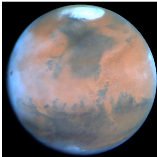
Полярные шапки Марса. Изображение с сайта http://www.astrolab.ru/cgi-bin/manager2.cgi?id=39&num=1430
