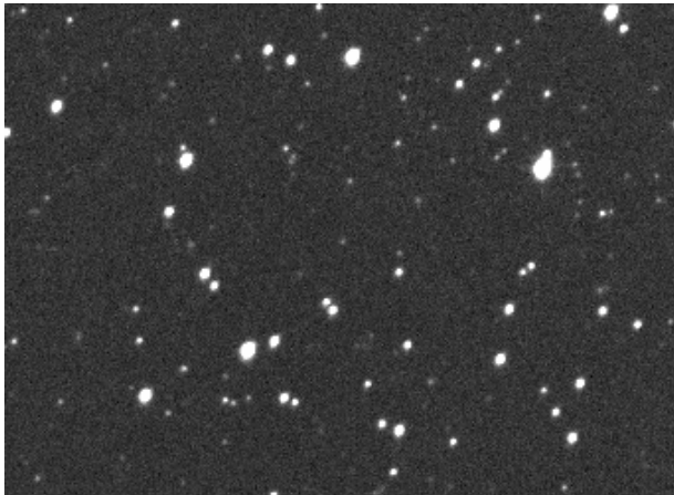
Астероид 2009 DD45 (в центре снимка). Изображение http://www.spaceweather.com с сайта http://www.astroalert.su
