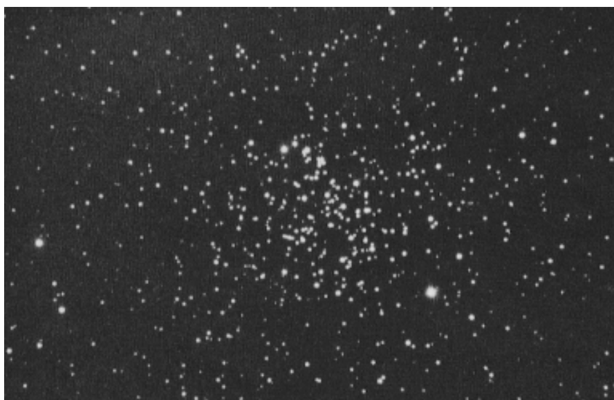
М67. Изображение с сайта tlgleonid.chat.ru/m.htm
