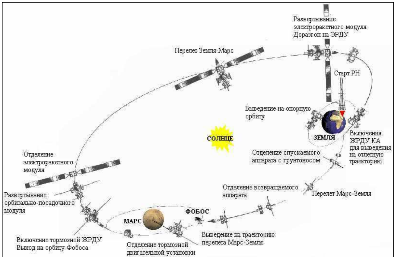
Схема полета аппарата «Фобос-Грунт». Изображение с сайта http://www.kiam1.rssi.ru/PHOBOS/
